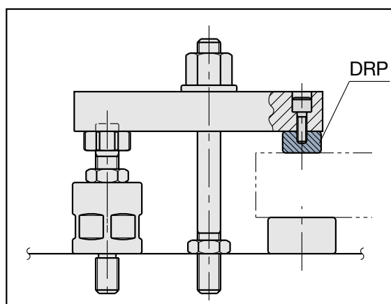
• Staffaggio del pezzo.
