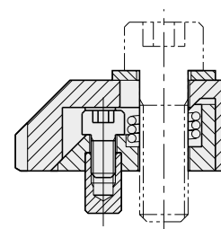
Sezione A-A
