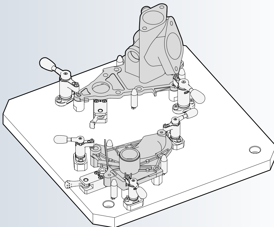
Attrezzatura con staffe pivotanti (Mini)
