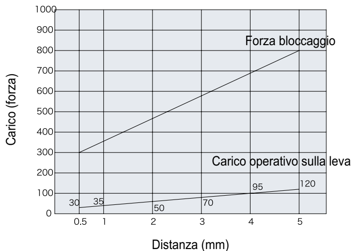
Staffa pivotante tipo 150
