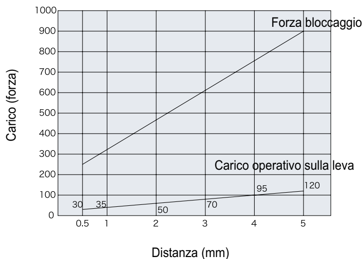
Modulo di spinta tipo 150
