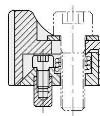
Sezione A-A
